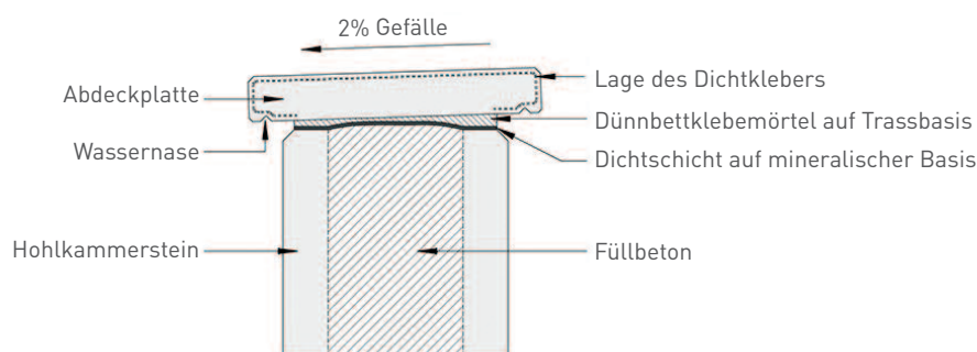
Abbildung 8: Skizze Dichtschicht und Abdeckplatte
